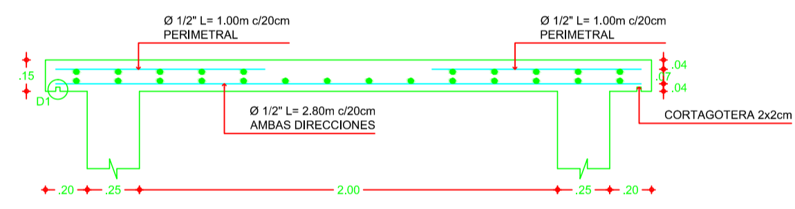
DETALLE LOSA NIVEL 2.65M Escala 1:20
