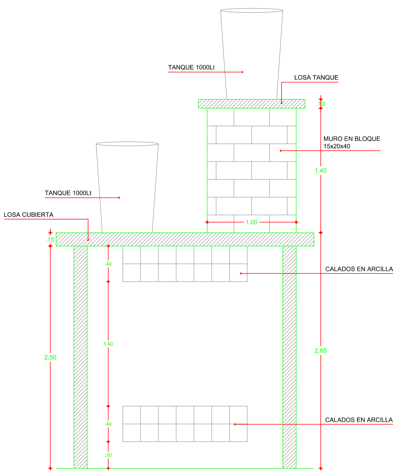
SECCION CASETA Escala 1:25
