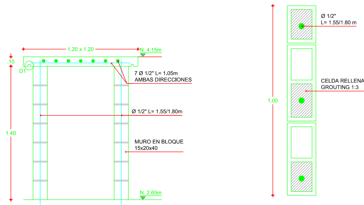
REFUERZO MURO EN BLOQUE 15x20x40 Escala 1:10
