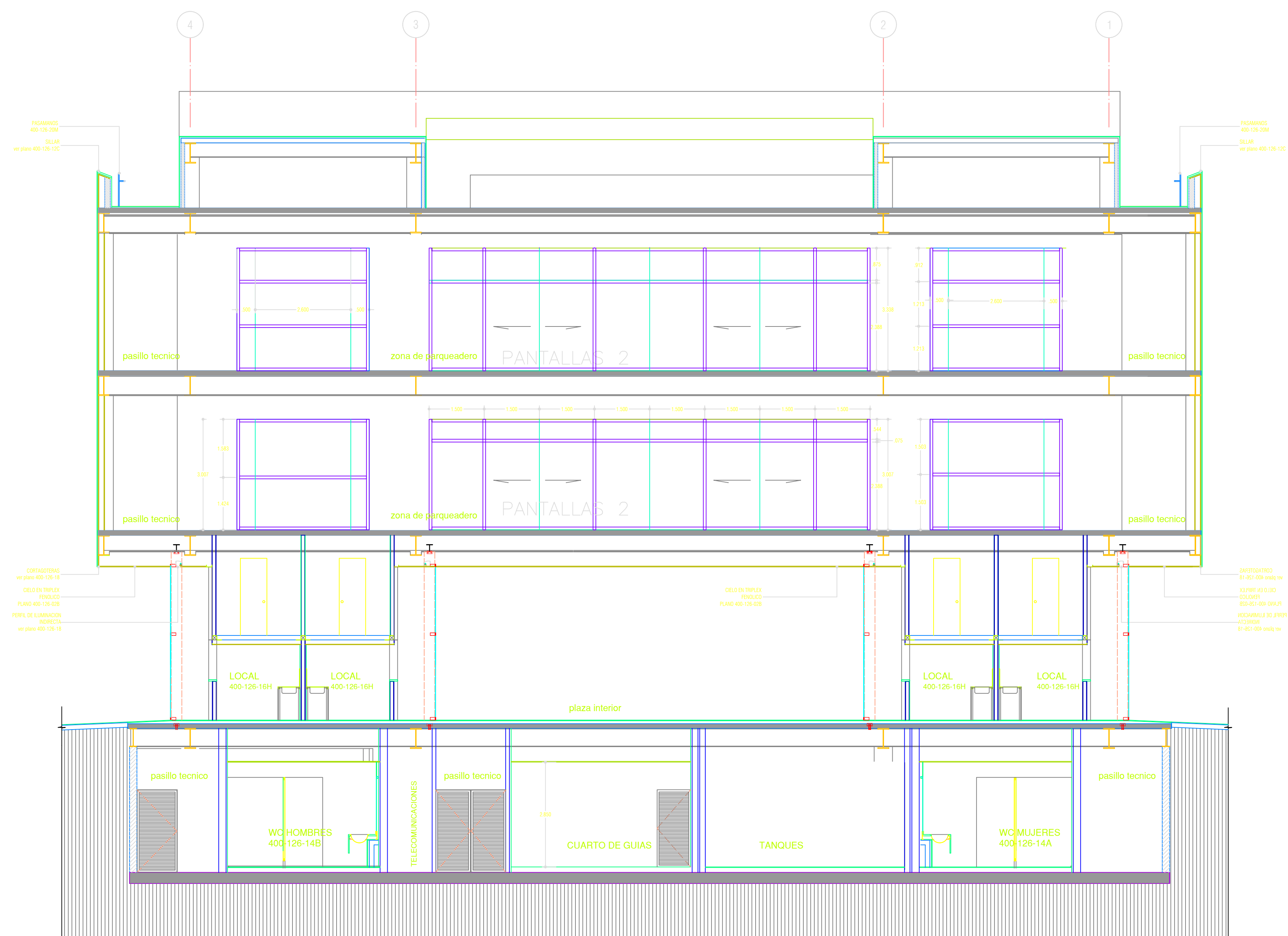
SECCIÓN 1-1 ESC 1:75
